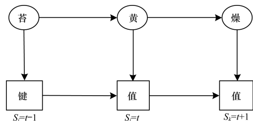
图 3 一阶 HMM 词性标注模型
