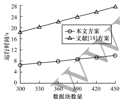
图3 证据验证阶段运行时间比较
