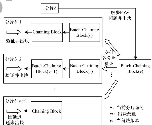
图1 Monoxide的出块方式
