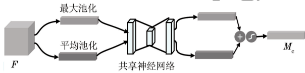
图 3 通道注意力模块示意图
