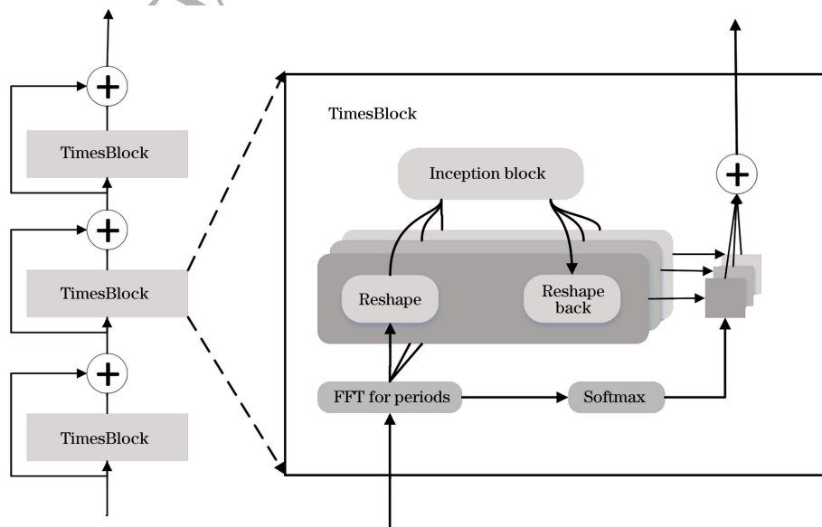
图 6 TimesNet 结构
