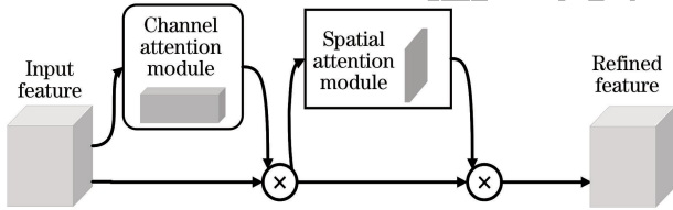
图 2 CBAM 整体架构
