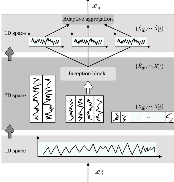
图 7 TimesBlock 过程图
