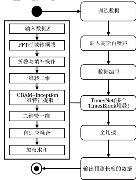
图 8 模型训练过程
