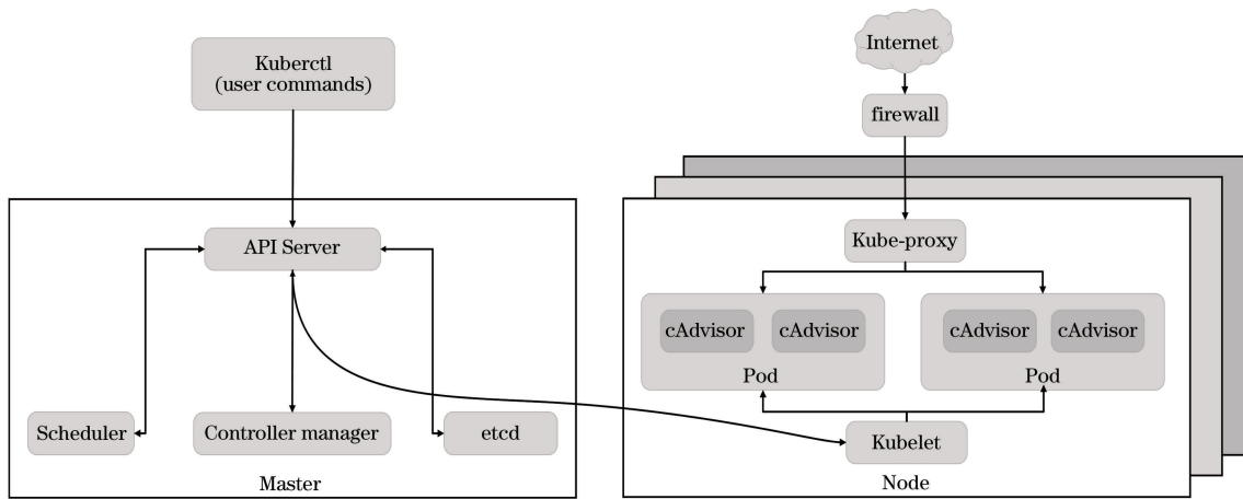
图 1 Kubernetes 总体架构
