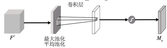
图 4 空间注意力模块示意图
